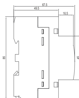
versiune 4 contacte
